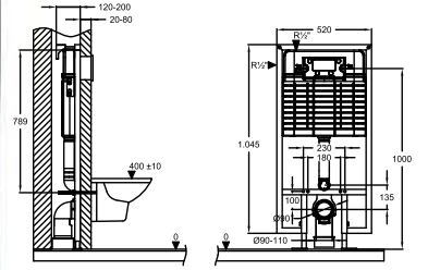
PROMICRO ALÇIPAN DUVAR ÖNÜ GÖMME REZERVUAR
