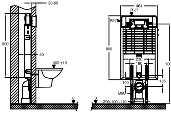
PROMICRO TUĞLA DUVAR İÇİ GÖMME REZERVUAR
