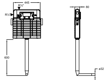
PROMICRO HELA TAŞLARI KLOZETLER İÇİN GÖMME REZERVUAR
